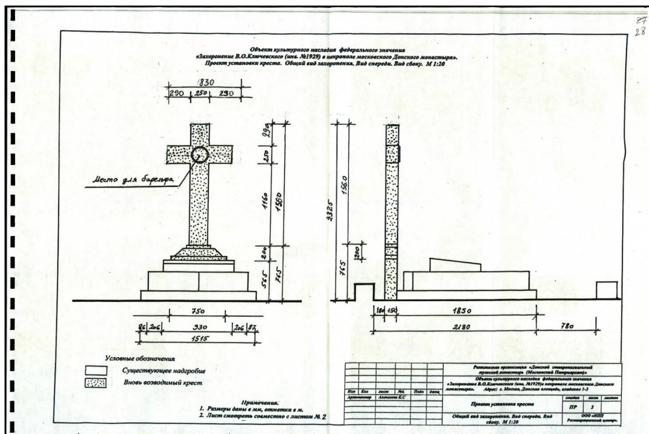
Копия чертежа из научно-проектной документации по установке креста
